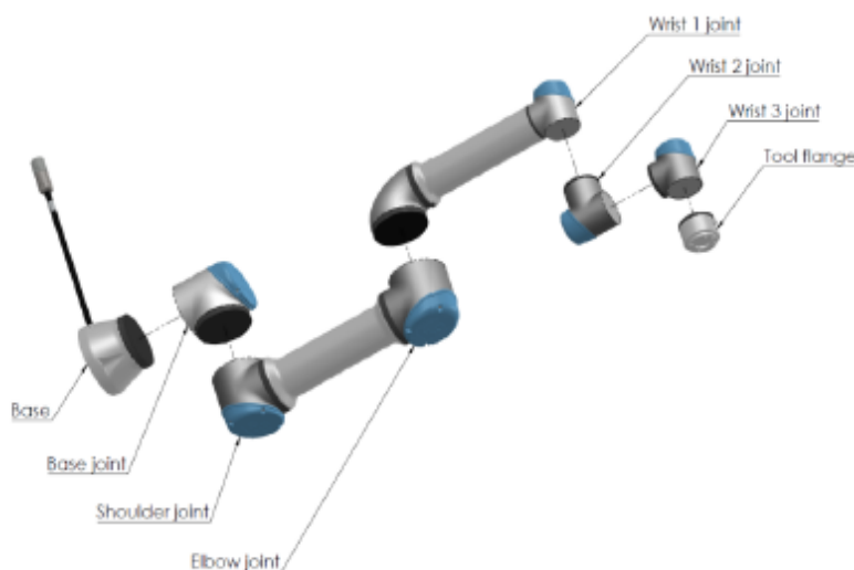
Robotarmens hovedkomponenter.
